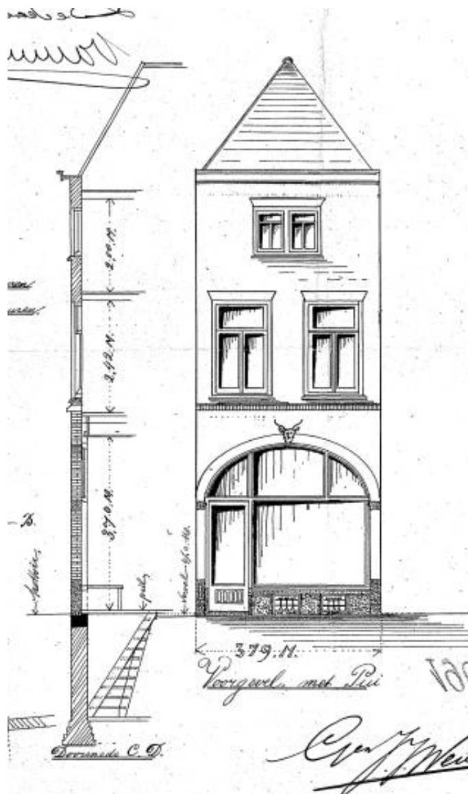
Bouwtekening met voorgevel uit 1906.
