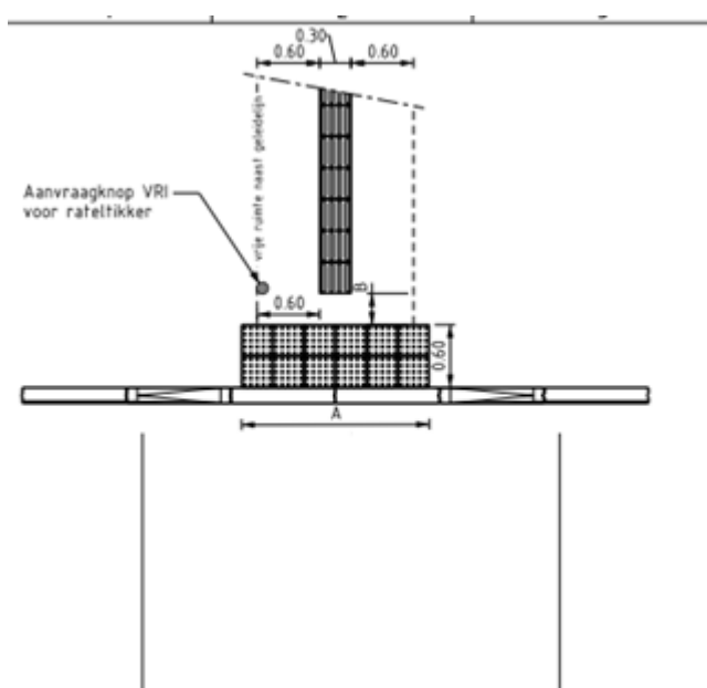
Figuur 18 Trottoirverlaging (Gemeente Nijmegen, Standaard Detailboek)
