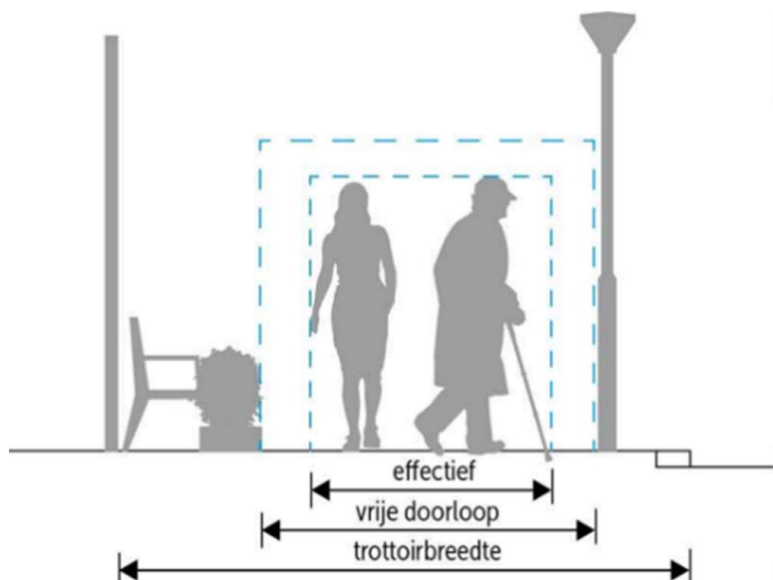
Figuur 3 Schematische weergave van de verdeling van de vrije en effectieve doorloopruimte (CROW, 2023)
