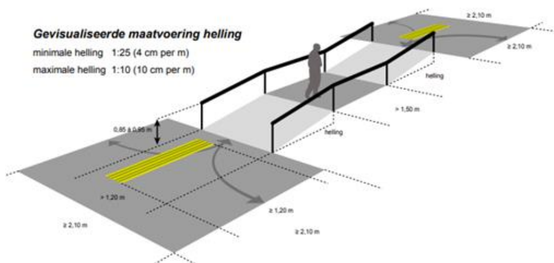
Figuur 21 Gevisualiseerde maatvoering helling (Gemeente Nijmegen)
