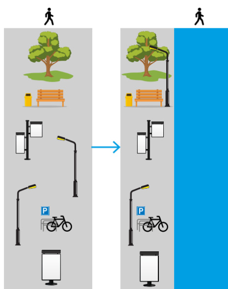
Figuur 2 Duidelijke obstakelvrije doorloopruimte creëren
