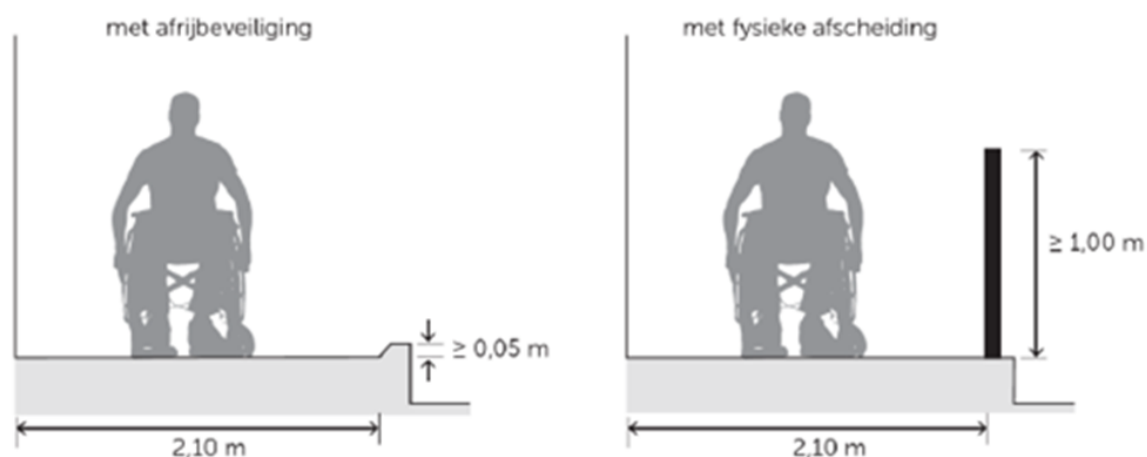
Figuur 17 Afmetingen valbeveiliging (CROW, 2025a).
