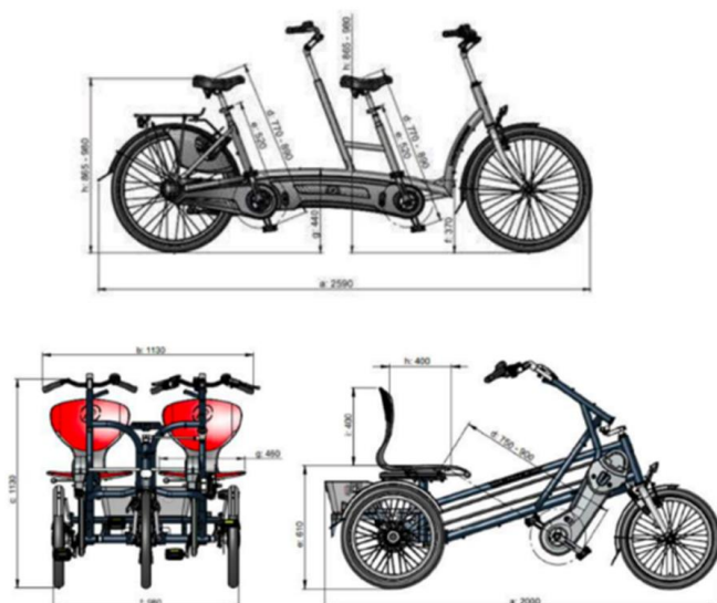
Figuur 15 Tandem en duofiets met afmetingen (CROW, 2024)
