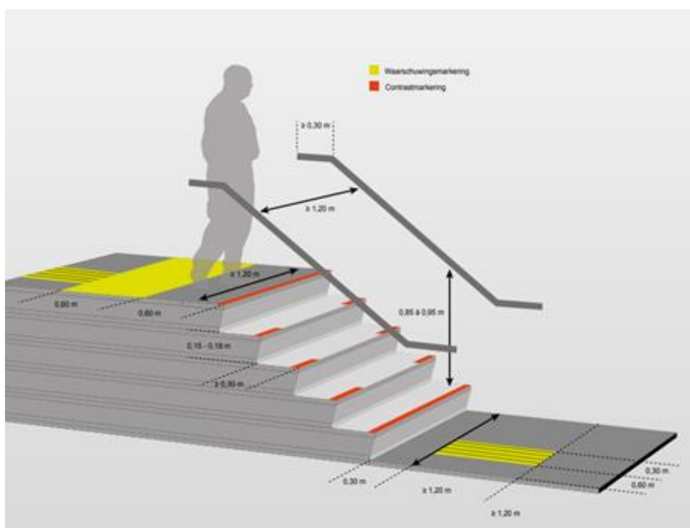
Figuur 19 Gevisualiseerde maatvoering van een trap (gemeente Nijmegen)
