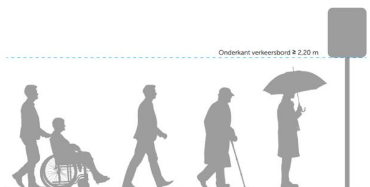
Figuur 4 Minimale vrije hoogte in de openbare ruimte (CROW, 2023)
