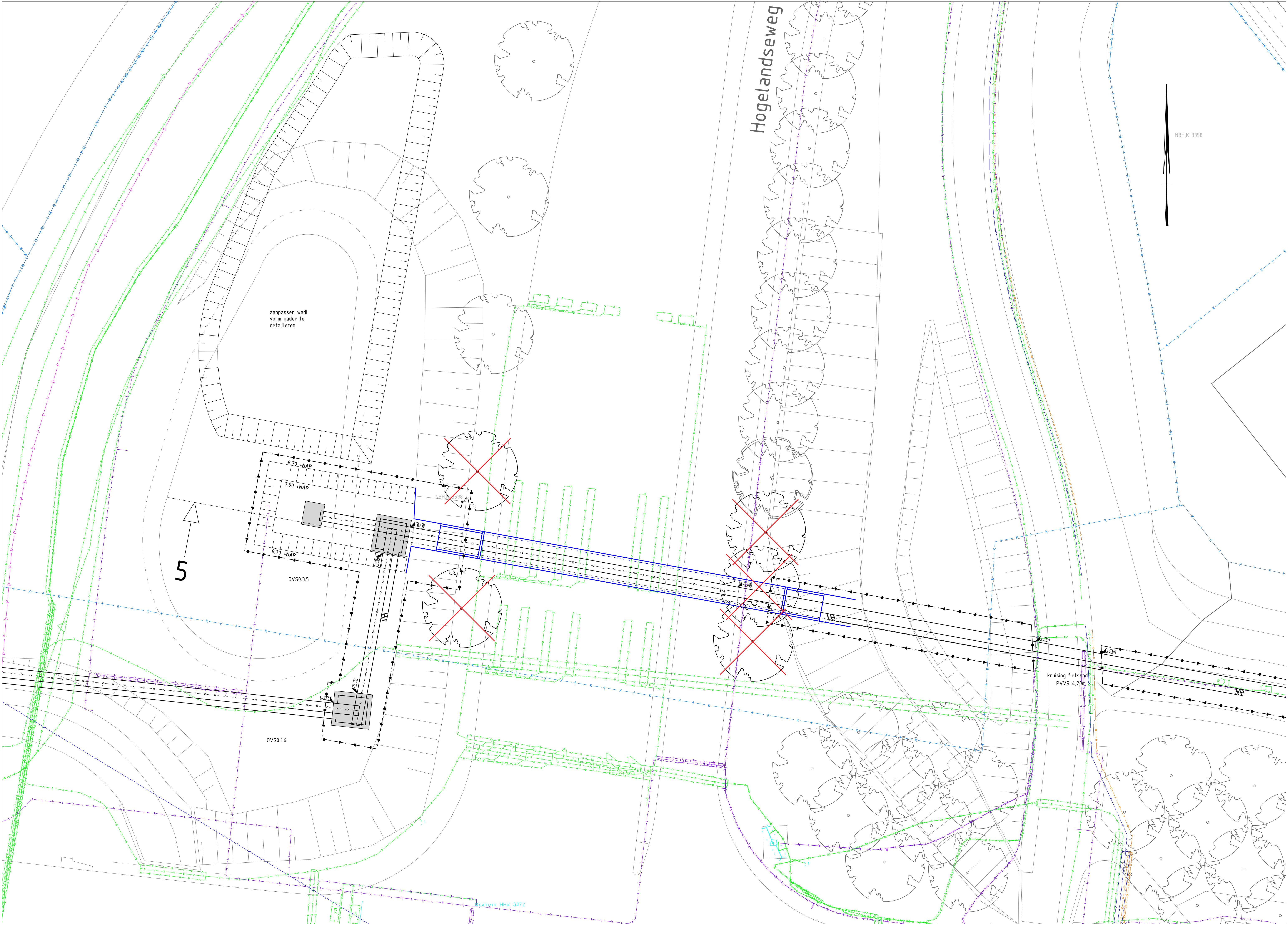
Detail 3 schaal 1:200
