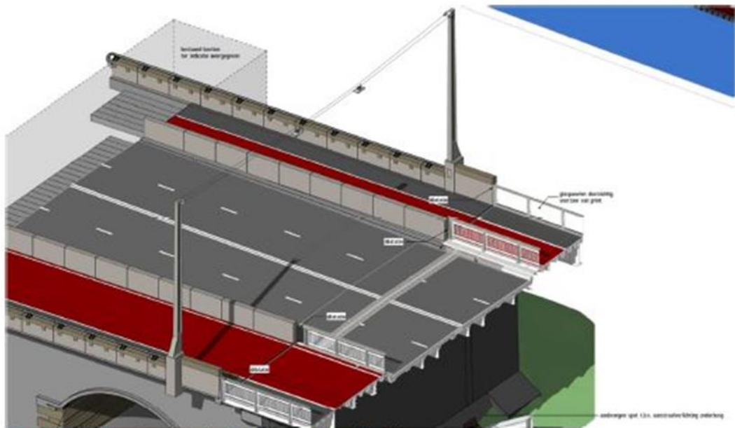
Figuur 25: Lichtmasten – principe t.p.v. bestaande landhoofden
