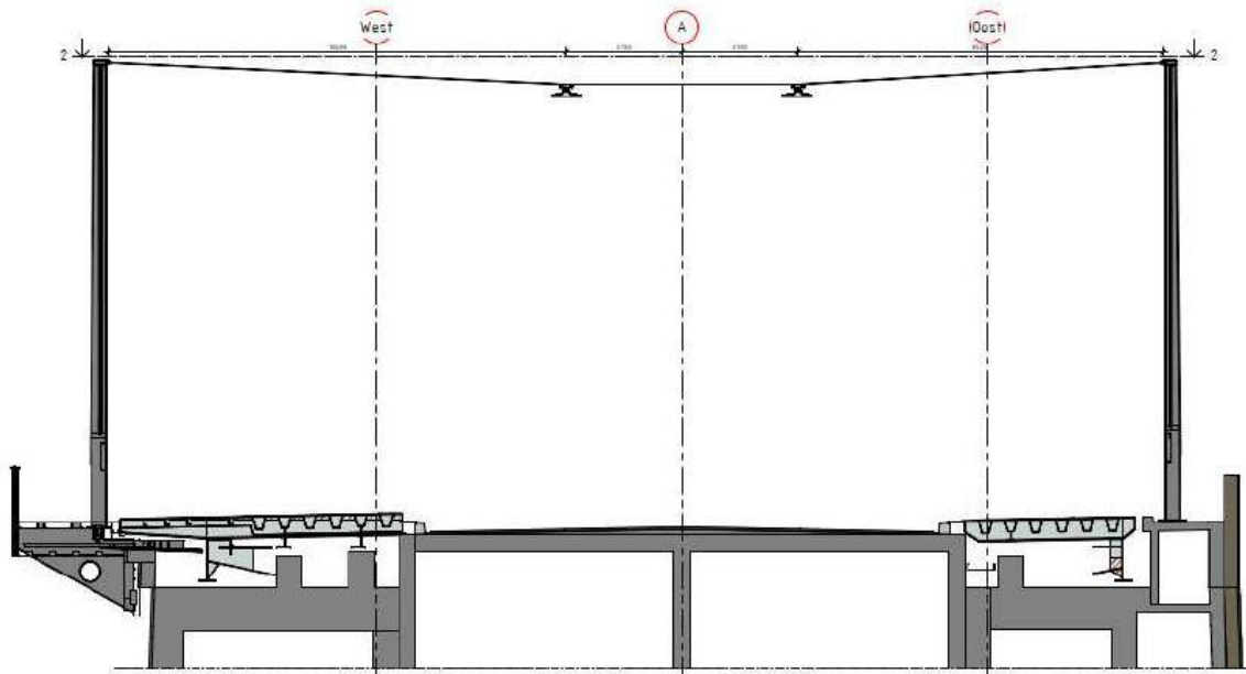
Figuur 6: Dwarsaanzicht verlichting aanbrug
