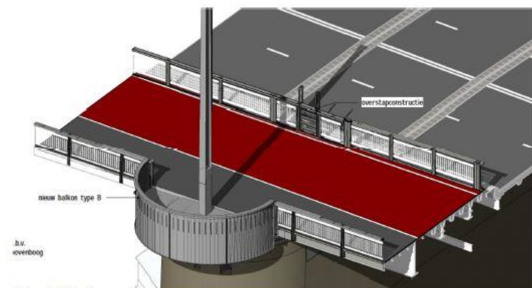
Figuur 21: Principe overstapvoorziening
