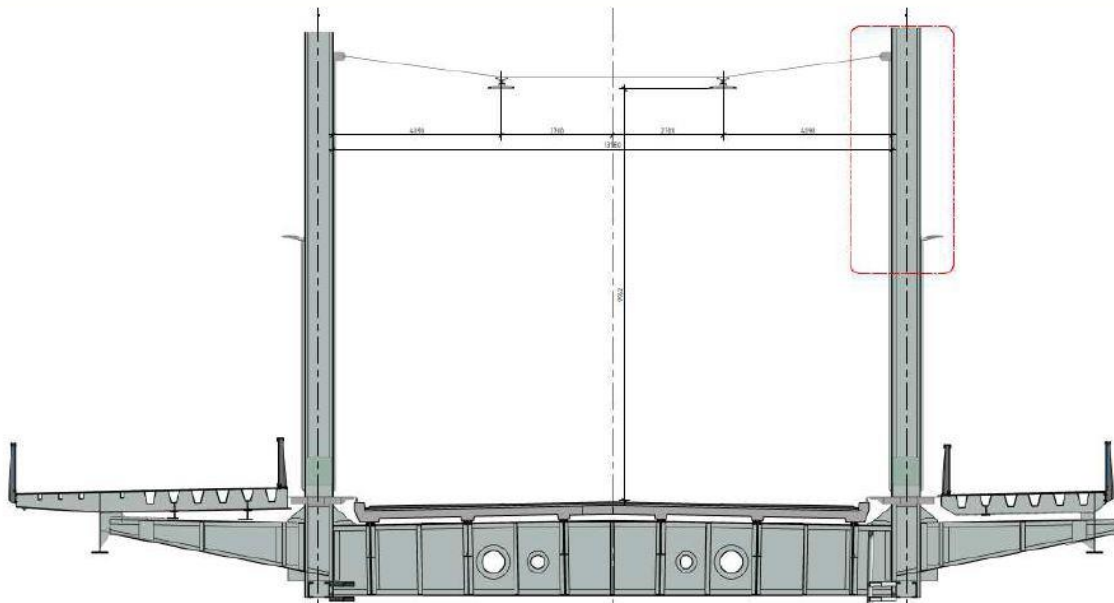
Figuur 4: Dwarsaanzicht verlichting hoofdo overspanning
