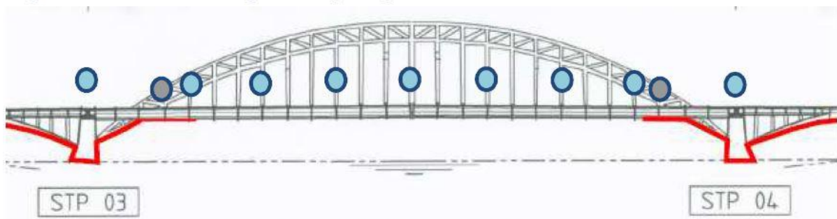
Figuur 3: Armaturen gelijk aan de hangers, tussenruimte van 2 hangers
