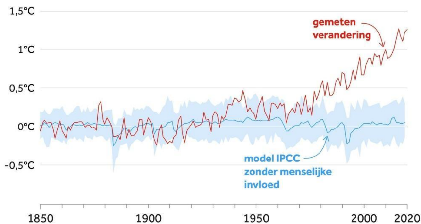
Figuur 1: Trent opwarming van de aarde met/zonder menselijke invloed op basis van bevindingen IPCC. 4
