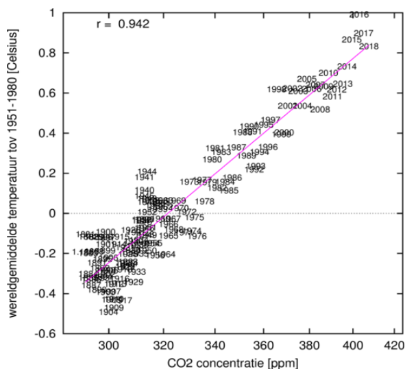
Figuur 2: wereldgemiddelde temperatuur (NASA/GISTEMP) uitgezet tegen de CO 2 concentratie. 6
