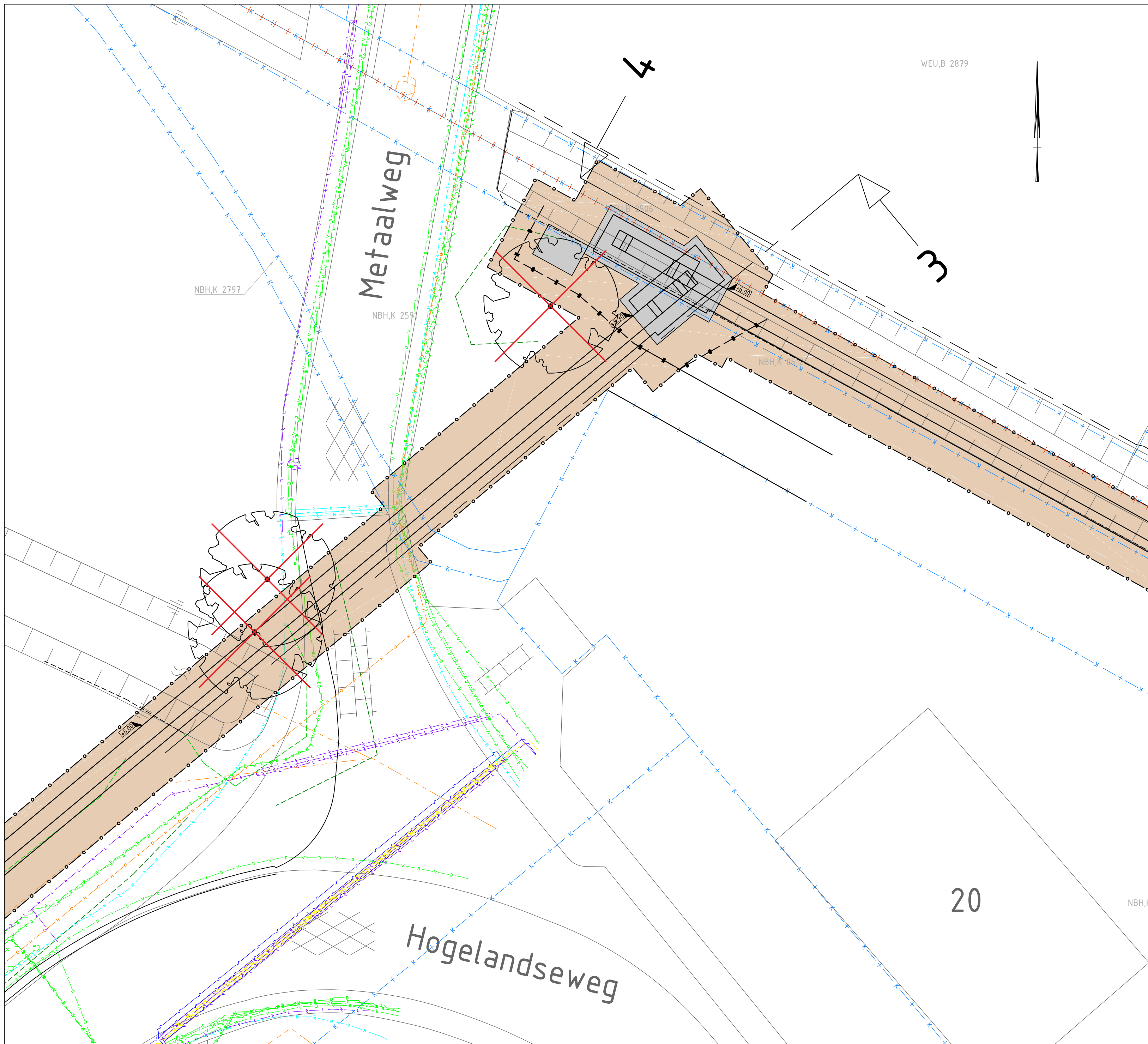
Detail 2 schaal 1:200
